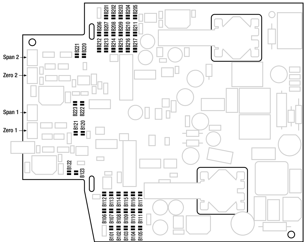
Fig. 2. Position of the soldered jumpers B ... and the potentiometers «Zero» and «Span».
